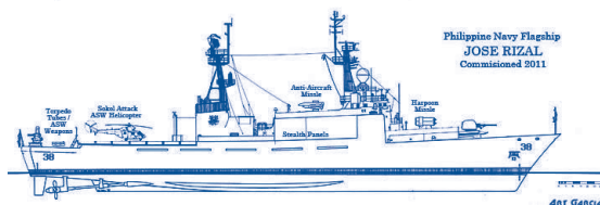
Plano de comparación de modificaciones hechas por la marina filipina. Fuente Philippine Navy.
